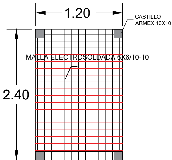
PLANTA DE CIMENTACIÓN
